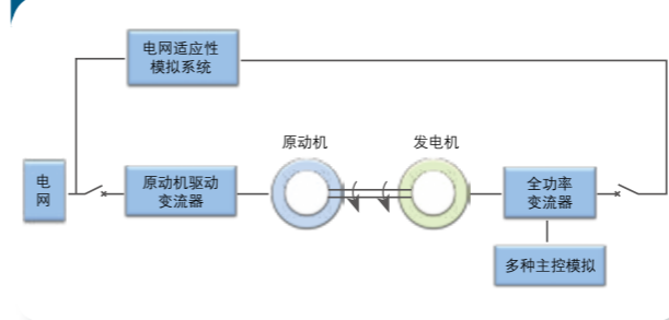
全功率机型试验系统示例
