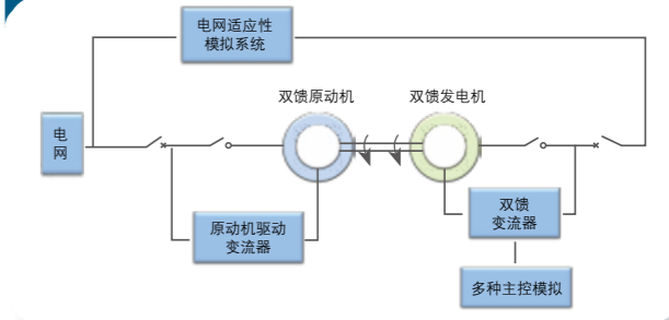
双馈机型试验系统示例
