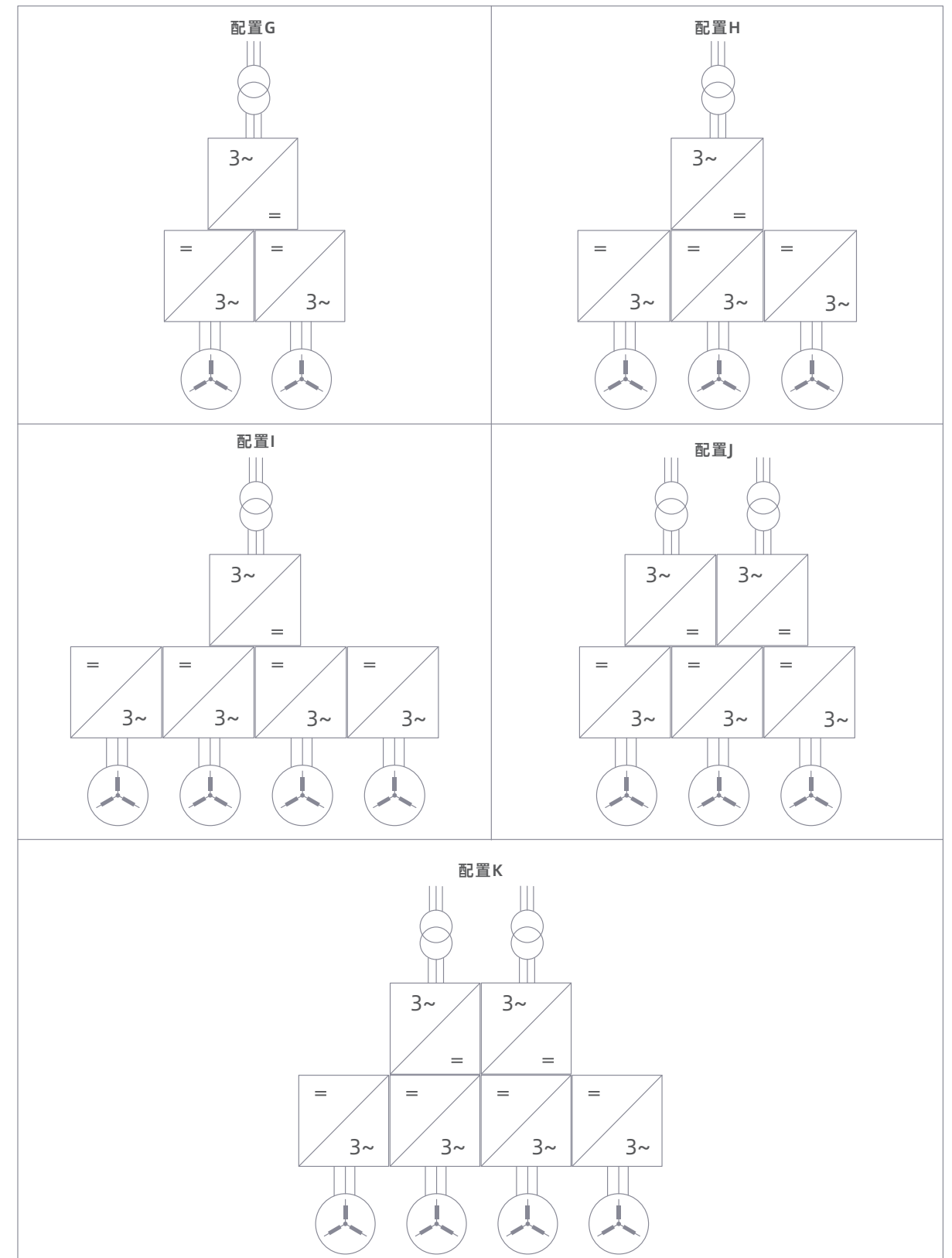
多传动系统配置示例
