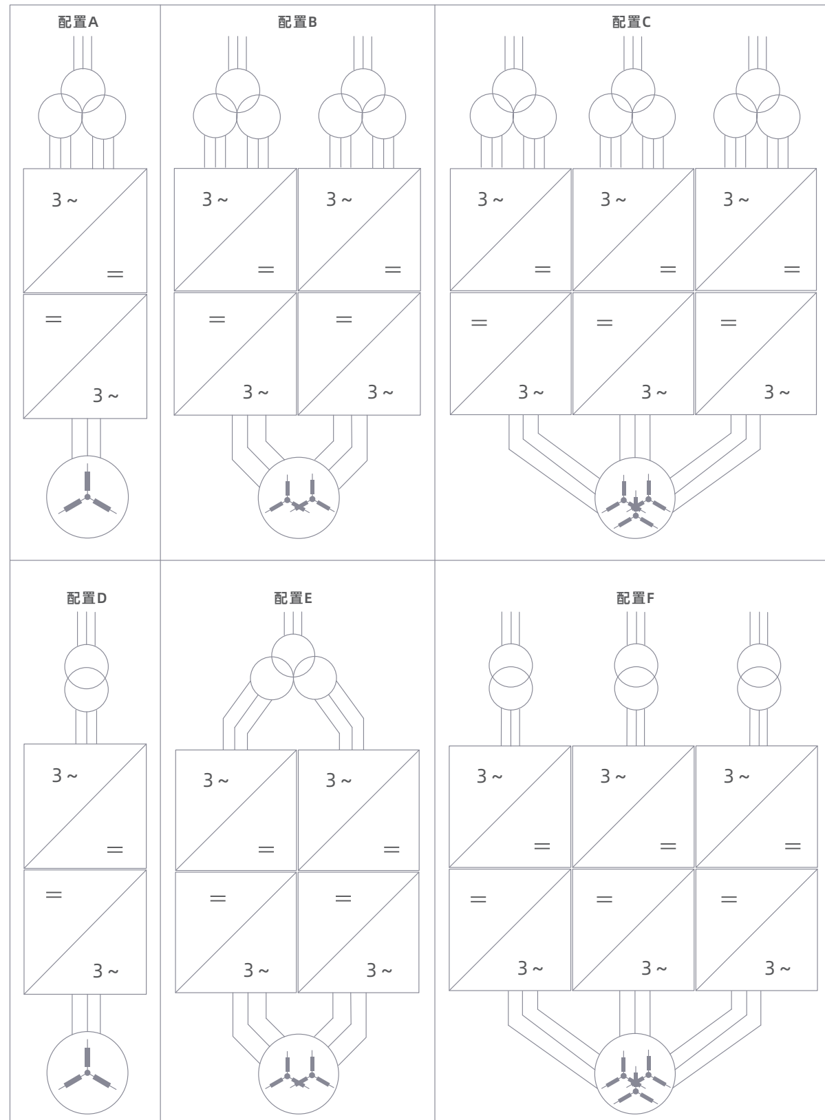
单传动/并机系统配置示例
