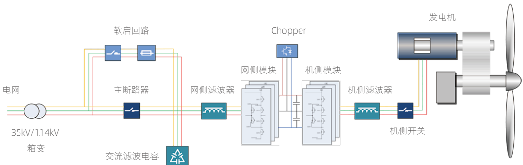
900V/950V/1140V全功率风力发电系统结构图
