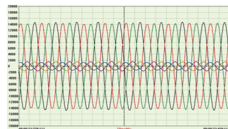
(补偿后-改善电网电压不平衡度很小)
